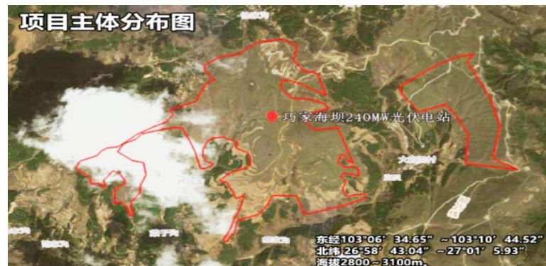
云南省昭通市巧家县海坝240MW光伏电站分布图
